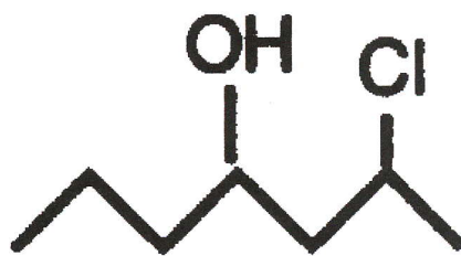
2-chloroheptanol
