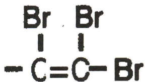
1,1,2-tribromoethene
